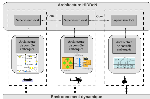
FIGURE 1 – L'architecture décisionnelle HiDDeN, supervisant l'équipe de véhicules
